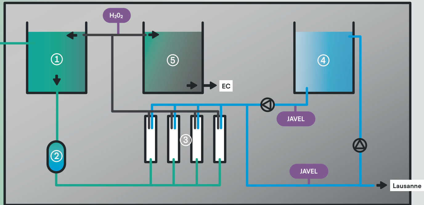
① Cuve eau brute ② Préfiltre ③ Ultrafiltration ④ Cuve rétrolavage ⑤ Cuve eau sale
