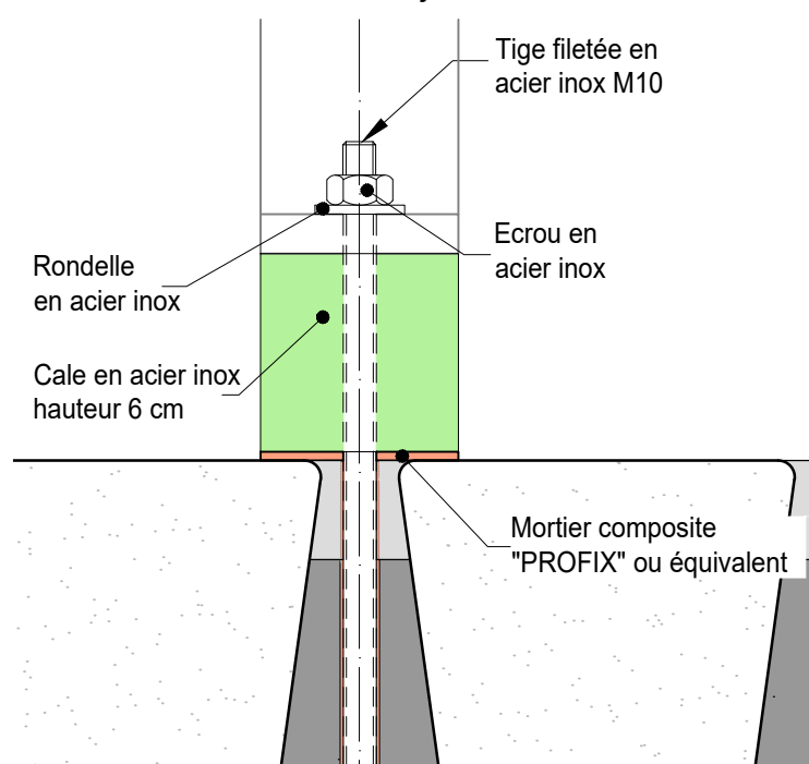
Détail de fixation
