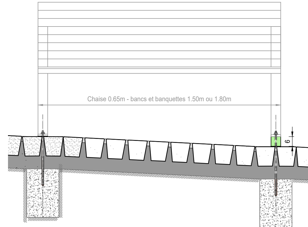
Chaise 0.65m Bancs 1.50m et 1.80m
