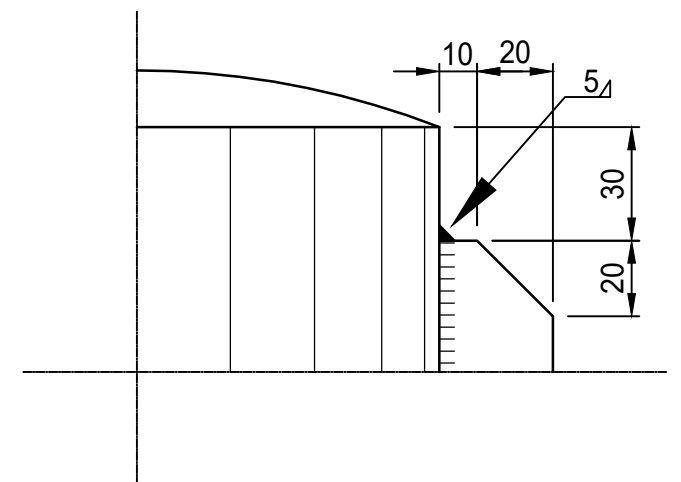
Détail 1:2
