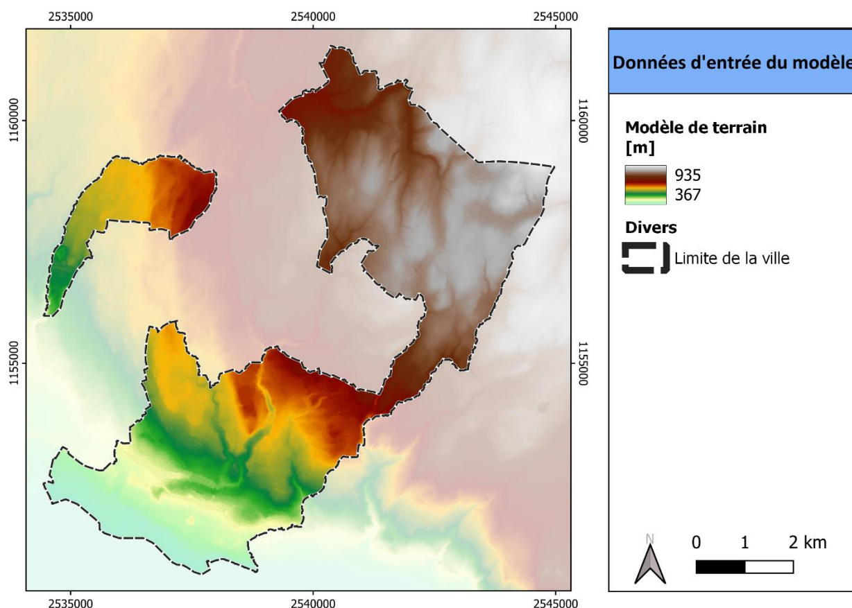
Fig. 1: Modèle numérique de terrain
