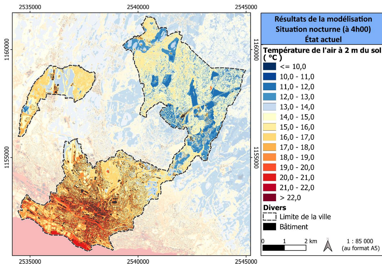
Fig. 5: Champ de température nocturne près du sol à Lausanne
