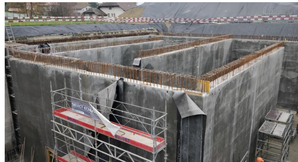
Construction de la nouvelle cuve
