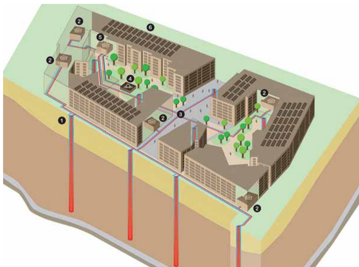
Concept énergétique des Plaines-du-Loup : 1. Sondes géothermiques à 800 mètres de profondeur, 2. Chaufferies 3. Réseau énergie de liaison entre les sondes 4. Récupération de chaleur sur les eaux usées 5. Chaufferie pour la récupération de la chaleur des eaux usées. 6. Panneaux solaires photovoltaïques.
