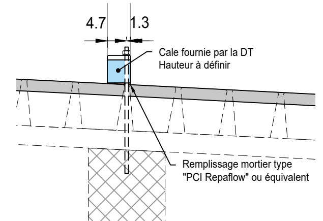
Calage sur surface perméable
