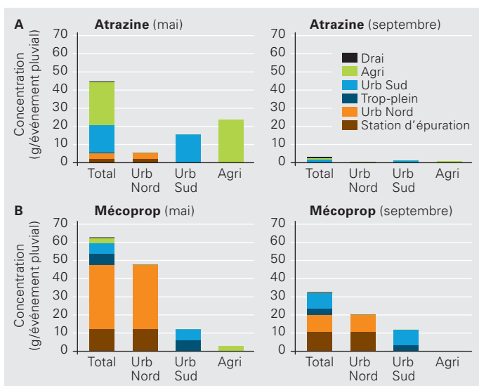
Fig. 3 : Comparaison des charges d'atrazine (A) et de mécoprop (B) dans six stations de mesure différentes (cf. Fig. 1) pendant une pluie de mai (60 mm de pluie) et une pluie de septembre (35 mm de pluie).
